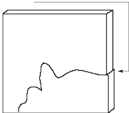
Figura 3: fractura de baja tensión
